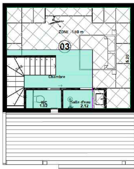
Comble
